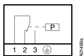
Anschluss als Sicherheitsdruckbegrenzer (SDBFS)
