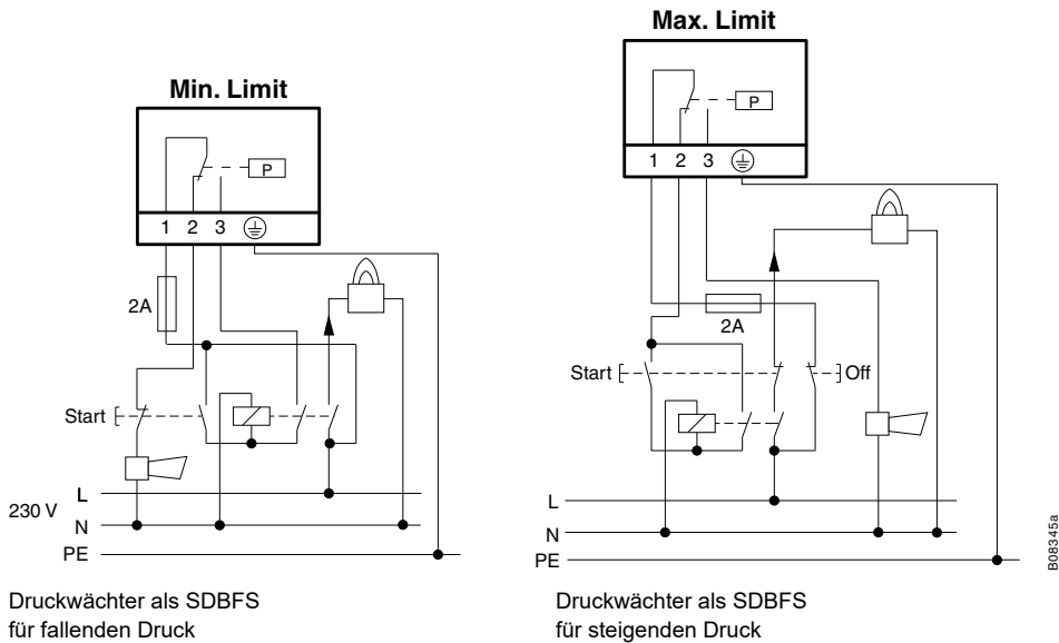
Anschluss als Sicherheitsdruckbegrenzer (SDBFS)
