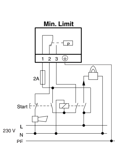
Druckwächter als Sicherheitsdruckbegrenzer für fallenden Druck
