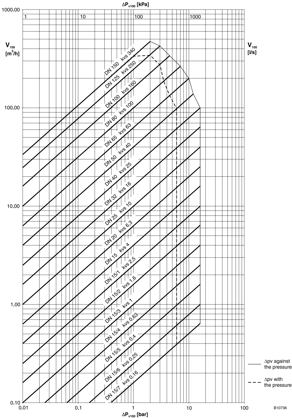
Diagramme de débit VUG
